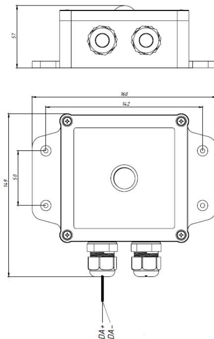
Рис.1 Габаритные размеры и схема подключения датчика
