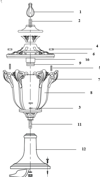
1 – балласт; 2 – резьбовое крепление; 3 – гровер; 4 – гайка; 5 – винты; 6 – верхняя крышка; 7 – каркас; 8 – стеклянный рассеиватель; 9 – патрон; 10 – ламподержатель; 11 – резьбовое крепление; 12 – постамент.
