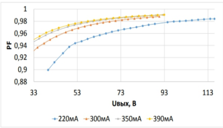
Зависимость коэффициента мощности от выходного напряжения
