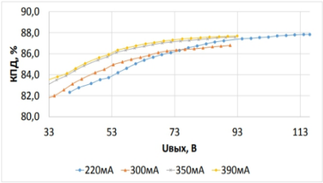
Зависимость КПД от выходного напряжения
