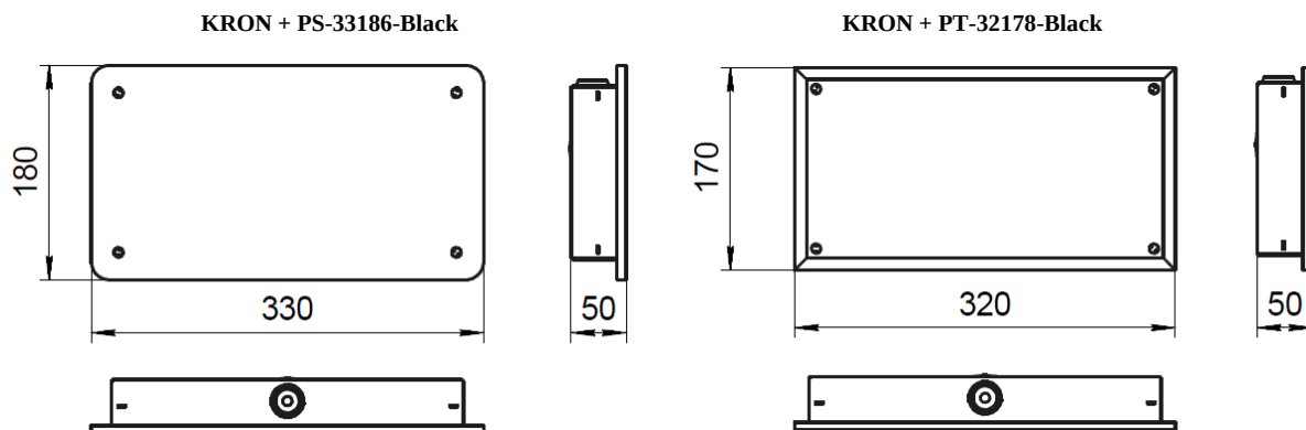
Рис. №2 Габаритный чертёж.
