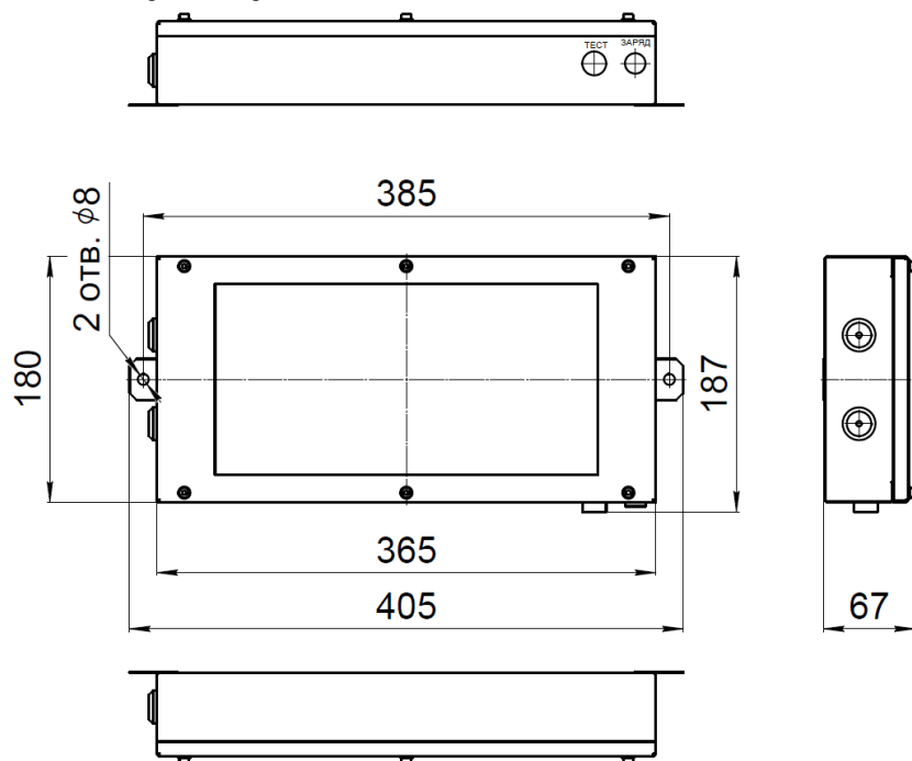
Рис. №2 Габаритный чертёж.
