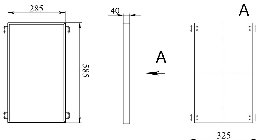
Рис.1 Габаритный чертеж.
