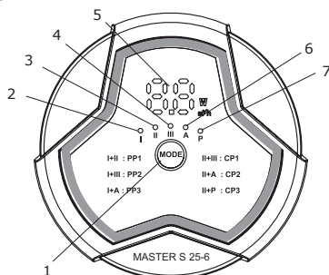
Рис. 12 Панель управления
