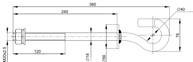
b) крюк монтажный / mounting hook / монтаждау ілмері В 20/240
