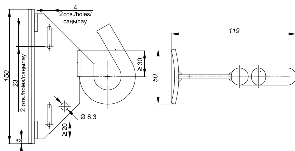
д) крюк монтажный / mounting hook / монтаждау ілмерінің SF 16
