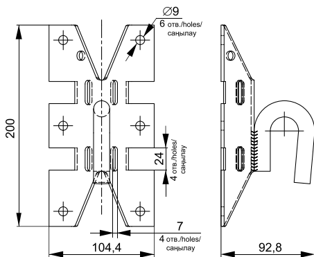
с) крюк универсальный / universal hook / әмбебап ілмері CS 16
