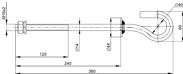
a) крюк монтажный / mounting hook / монтаждау ілмері В 16/240
