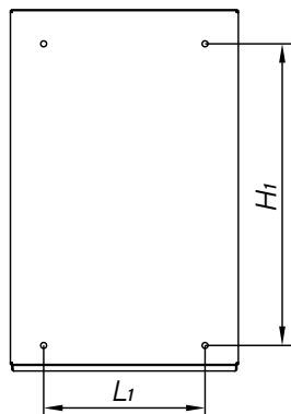
Вид сзади
