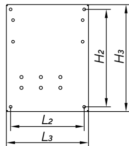
Панель монтажная
