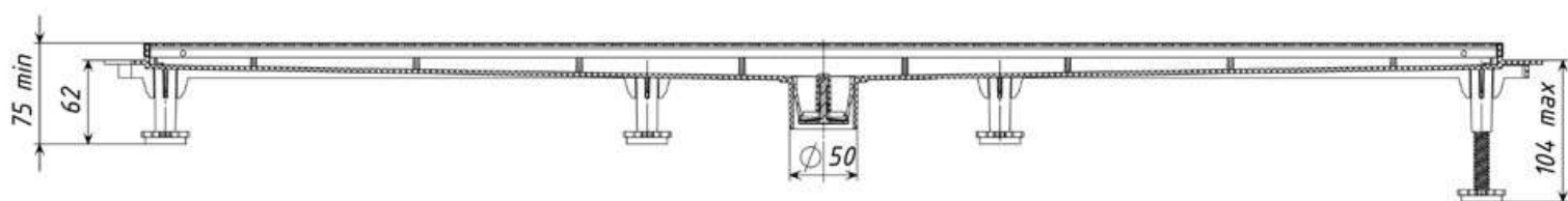
Вариант установки без затвора
