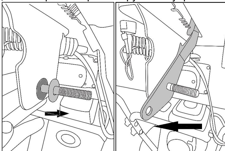
Рис. 11. Установка ручки
