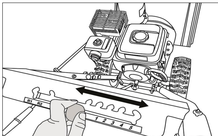
Рис. 44. Включение скорости
