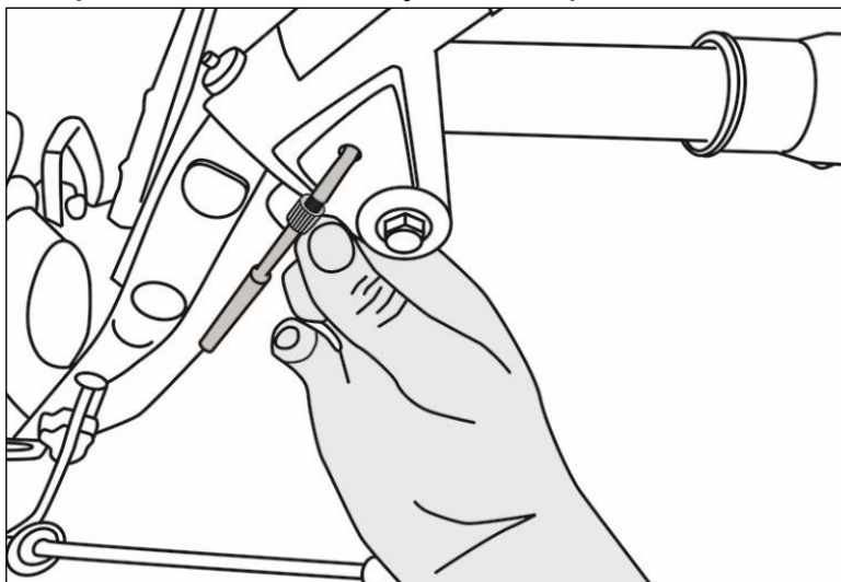
Рис. 8. Натяжка троса
