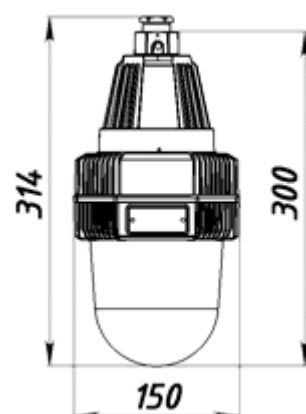
GLOBUS LED 15/25 D120 G Ex
