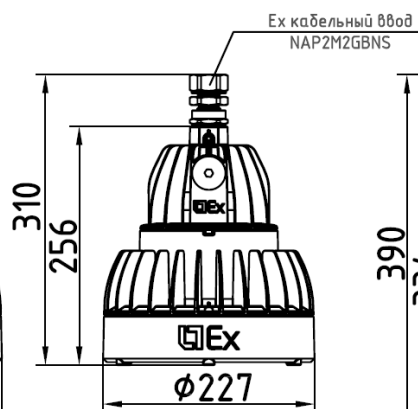
Globus LED D120 G Ex
