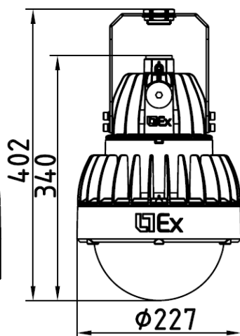
Globus LED D270 BT Ex
