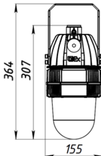
GLOBUS LED 15/25 D120 B Ex
