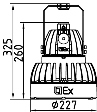
Globus LED D120 BT Ex
