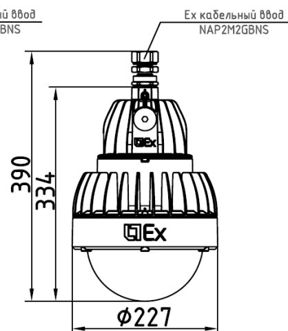
Globus LED D270 G Ex
