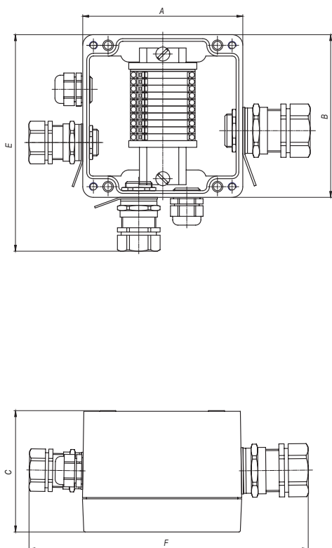
Рисунок 2. Модели PTB 404, PTB(i) 404
