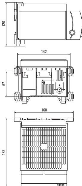
Рис. 1 Габаритные размеры обогревателя
