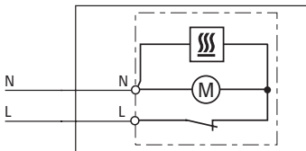
Рис. 2 Подключение обогревателя
