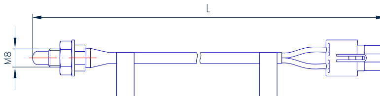
Рисунок 1 - Габаритные и присоединительные размеры датчика
