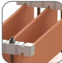
Шины располагаются вертикально для лучшего охлаждения
