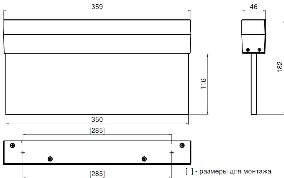
Рис. №2 Габаритный чертёж.
