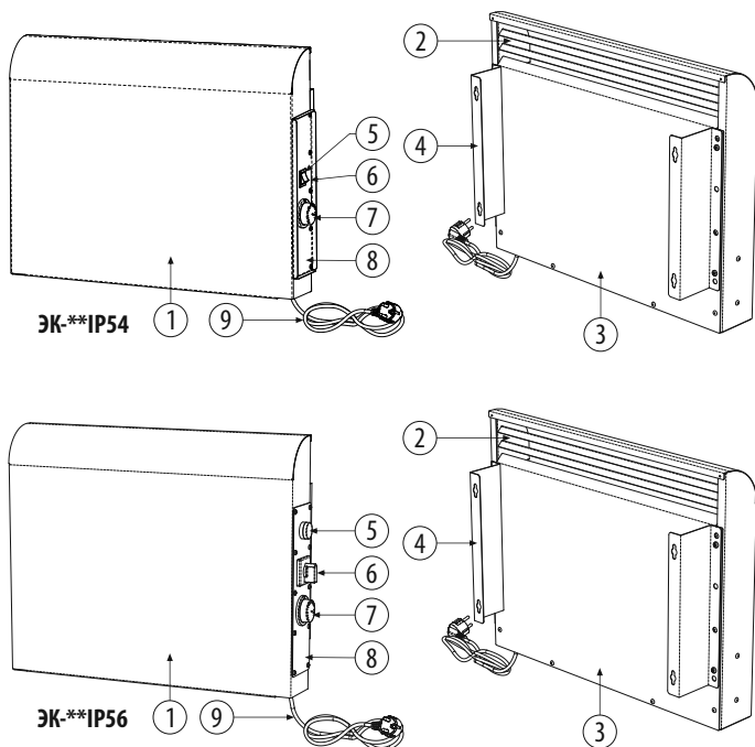
Рисунок 1. Внешний вид и элементы конструкции конвектора
