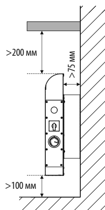
Рисунок 4. Размещение конвектора
