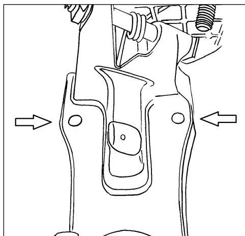
Рис.5 Крепление основания
