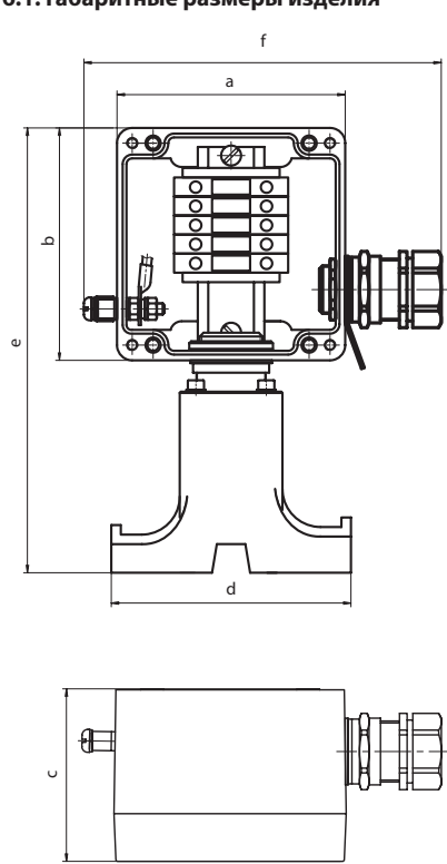
Рисунок 1. Серия РТВ 401
