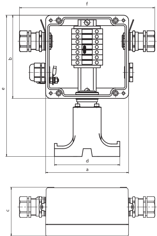
Рисунок 2. Серия РТВ 601
