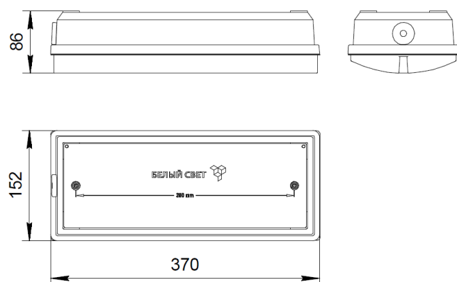
Рис. №2 Габаритный чертёж.
