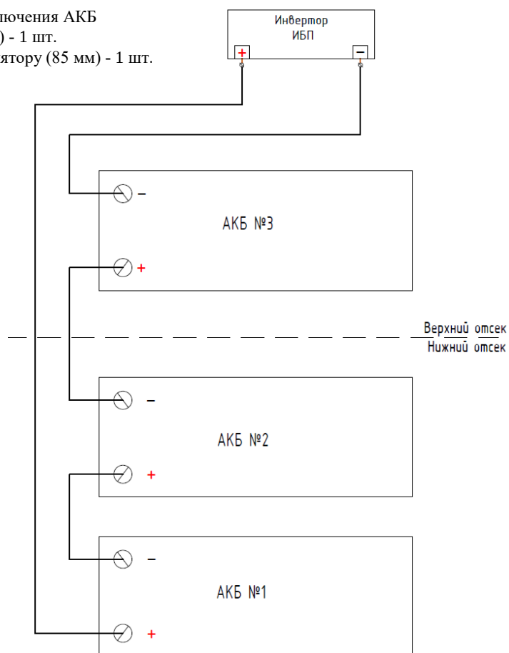
Рис. №2 Схема подключения аккумуляторных батарей.
