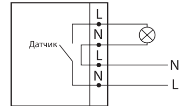
Рисунок 2. Схема подключения датчиков
