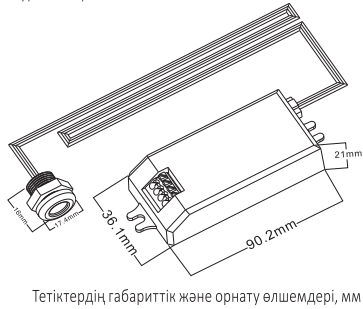
Тетіктердің габариттік және орнату өлшемдері, мм
