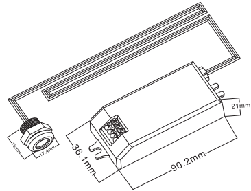
Рисунок 1. Габаритные и установочные размеры датчиков, мм
