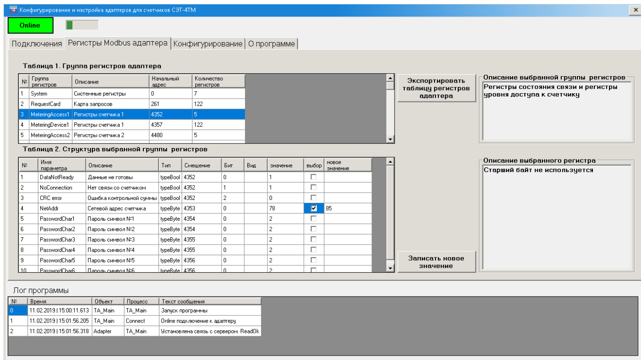
Рисунок 4 – Настройка параметров доступа и проверка связи со счетчиком.
