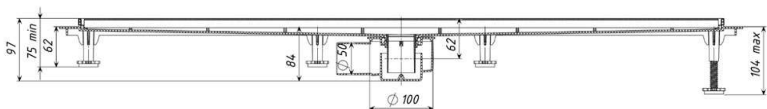
Вариант установки с гидрозатвором
