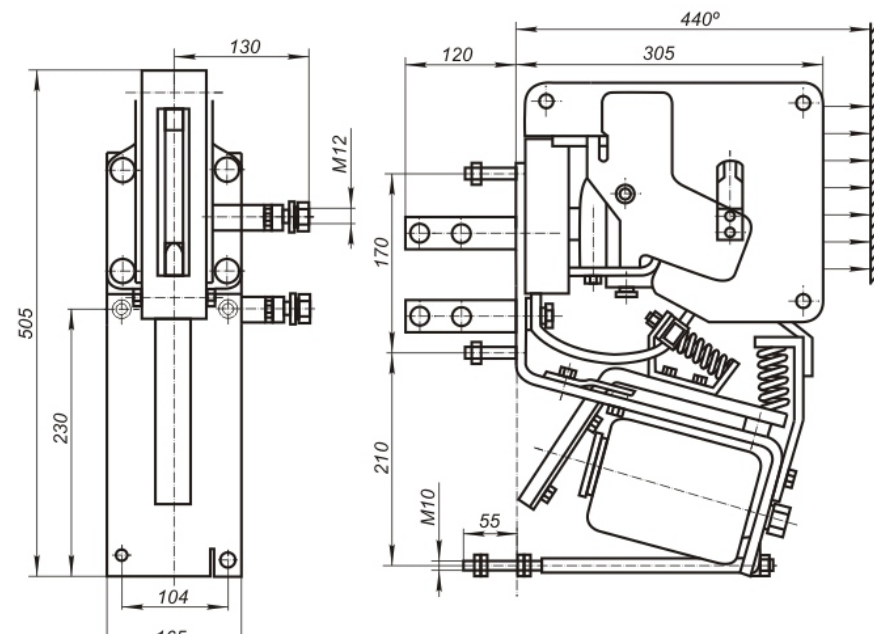
Габаритные размеры контакторов КПВ-605
