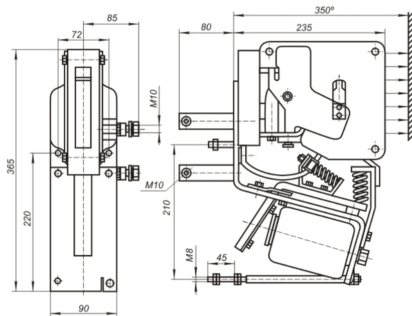
Габаритные размеры контакторов КПВ-604
