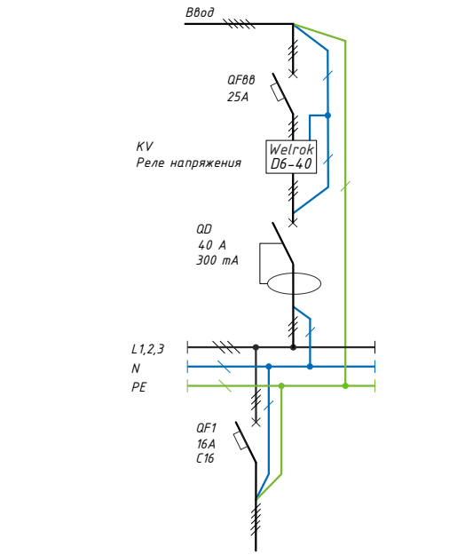
Схема 2. Вариант электрической схемы с трехфазной нагрузкой
