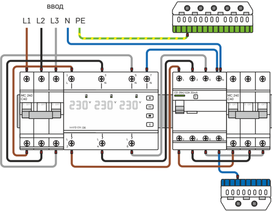
Схема 1. Монтажная схема
