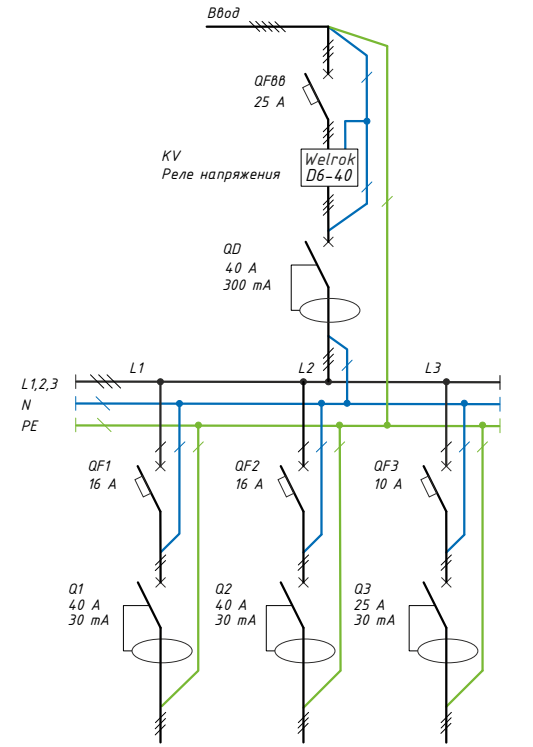
Схема 3. Вариант электрической схемы с тремя однофазными нагрузками
