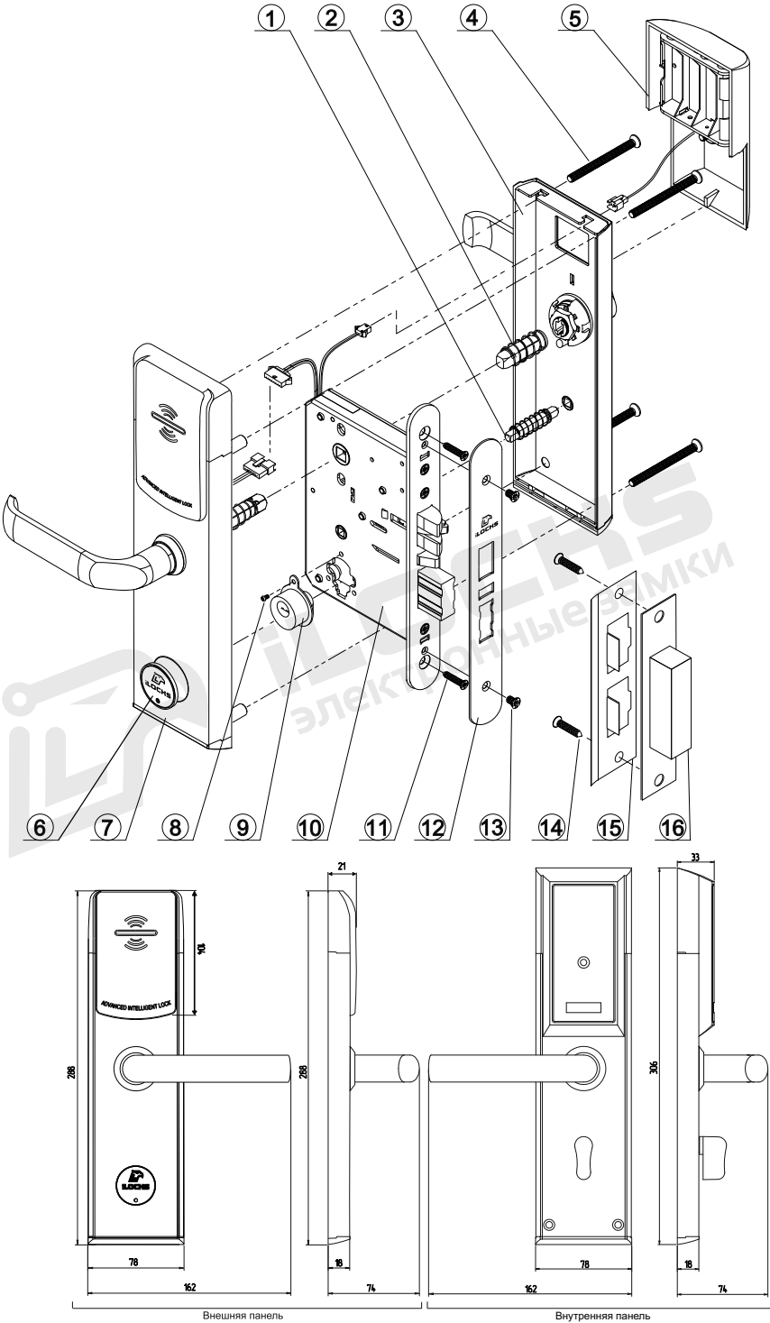
Рисунок №1 – Структурная схема (спецификация) замков типа iLOCKS IS8005AB3
