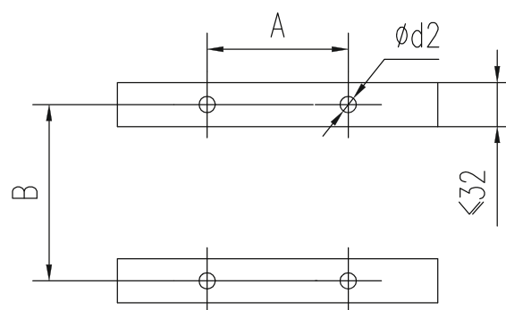
Габаритные и установочные размеры корзины выкатного типа
