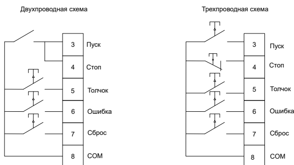
Рисунок 3.4 – Схемы подключения входов управления
