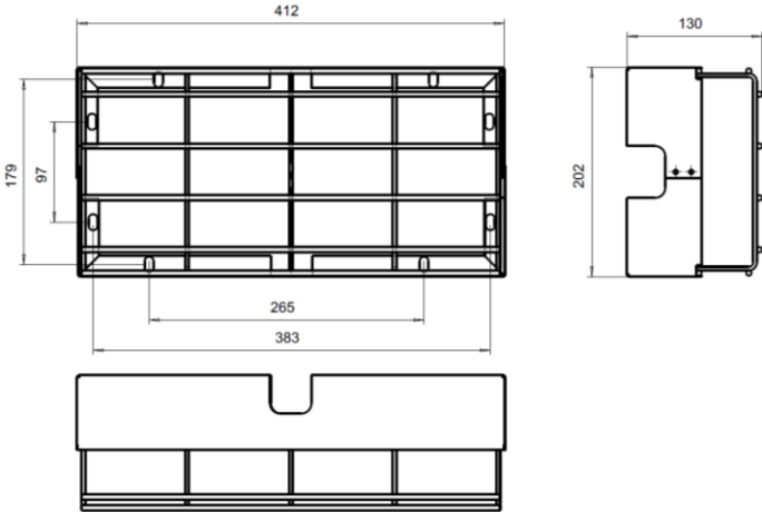
Рис. №3 Аксессуары. Решётка защитная BS-R-1 (а2333)
