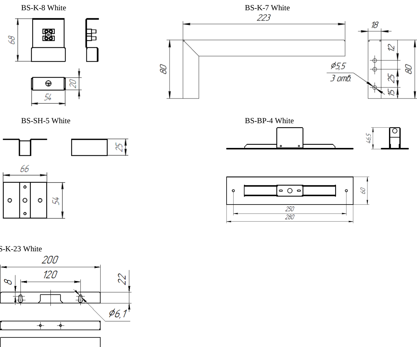
Рис. №3 Аксессуары
