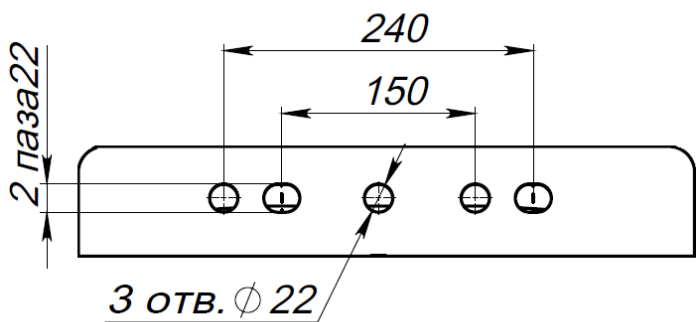
Монтажные отверстия
