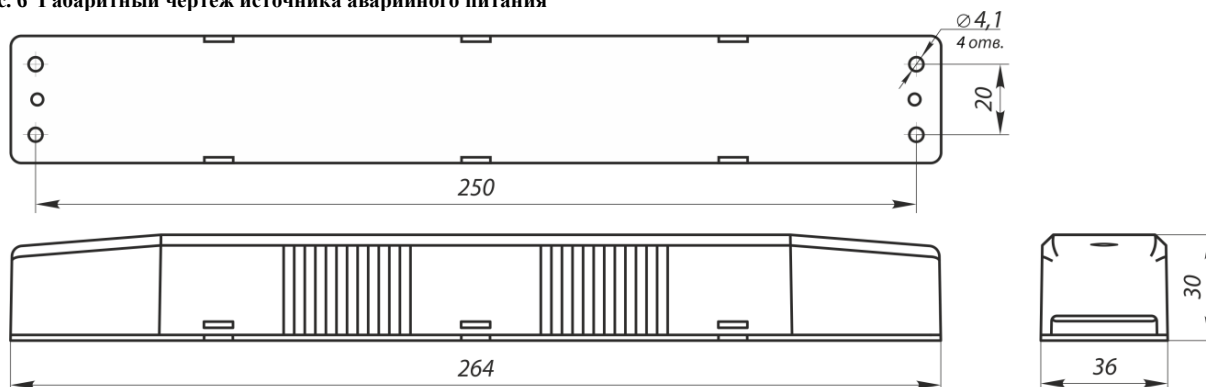
Рис. 6 Габаритный чертеж источника аварийного питания
