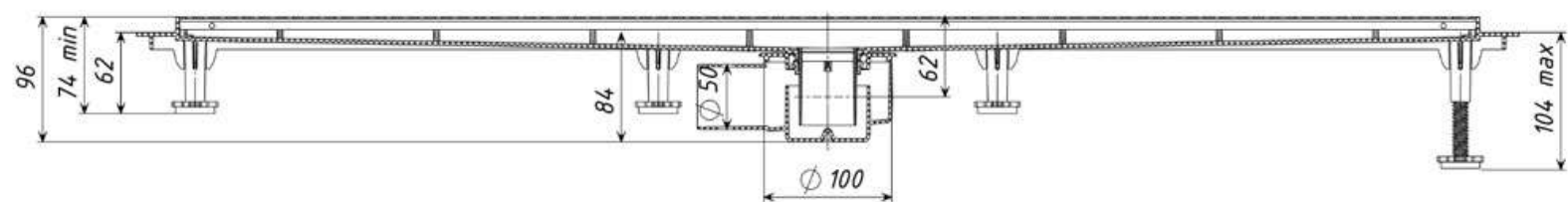
Вариант установки с гидрозатвором
