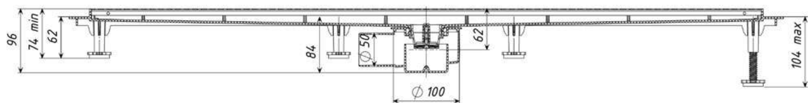
Вариант установки механического "сухого" затвора
