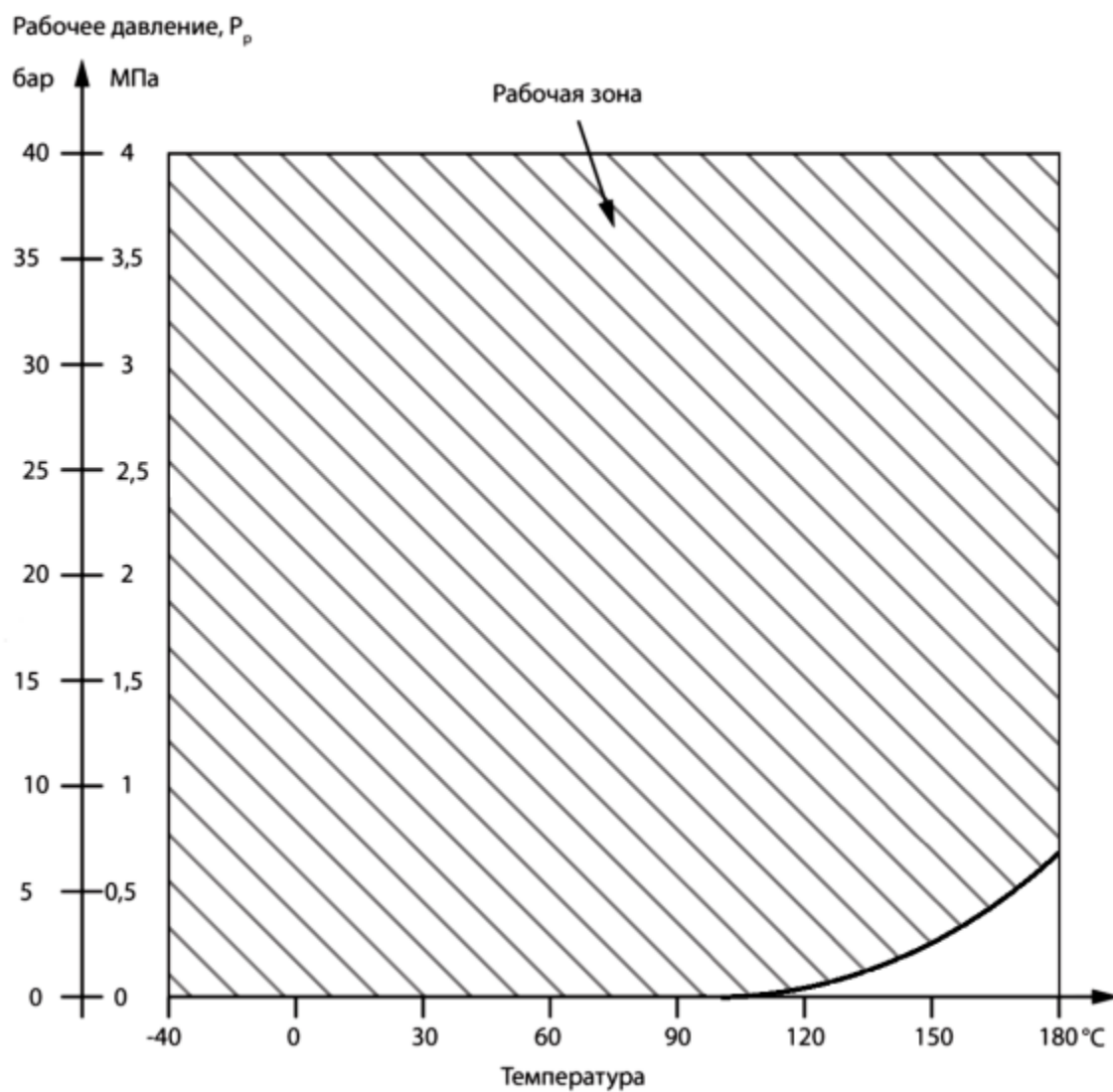
График Температура-Давление
