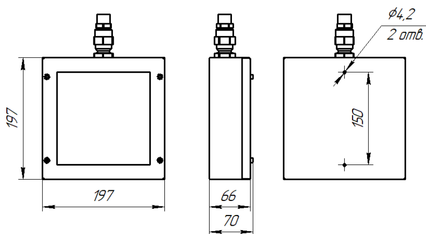
Рис. №2 Габаритный чертёж.
