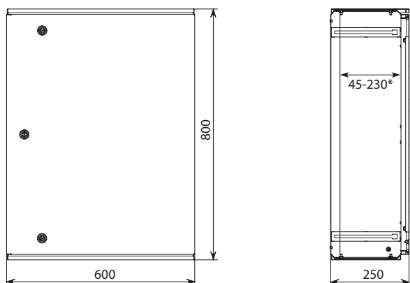
ЩМПг-80.60.25
