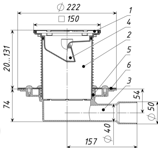
Рис. 1 ТП-510.1N-3000 Трап с незамерзающим запахозапирающим устройством
