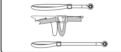
Рис. 7. Регулировка длины
