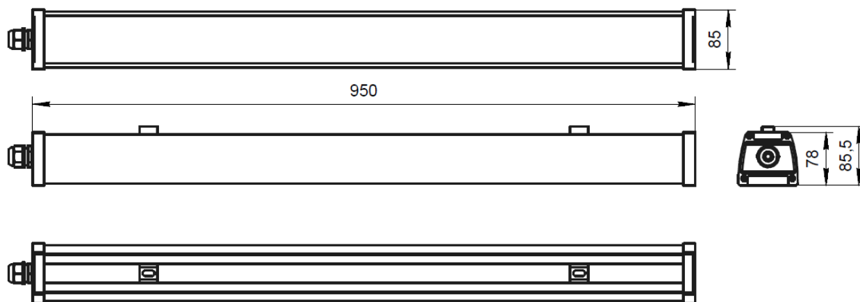
Рис. №2 Габаритный чертёж.
