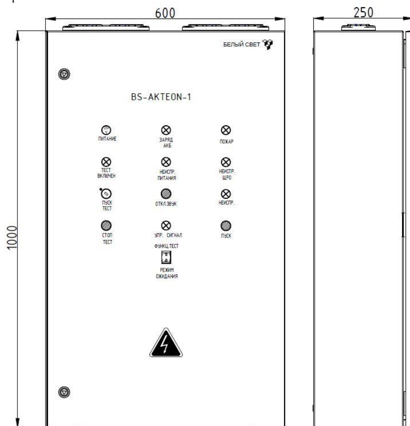
Рис. №2 Установочный чертёж.
