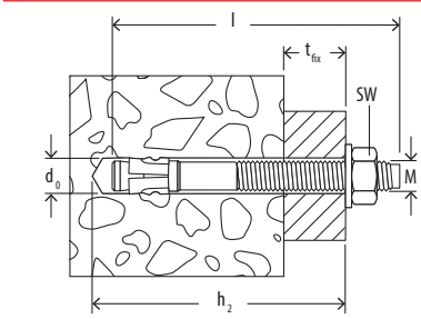
Анкерный болт FWA Plus
