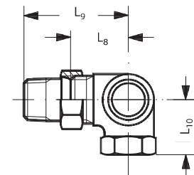
Угловой трехходовой клапан (правое исполнение)
