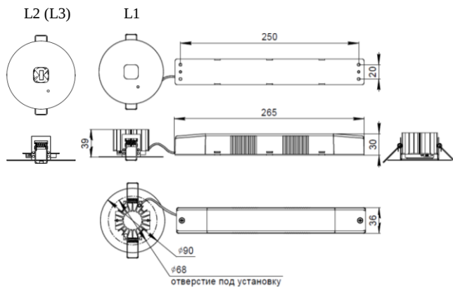
Рис. №3 Габаритный чертёж.
