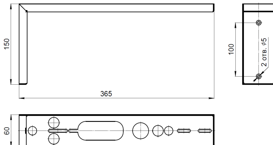
Рис. 3.2 Кронштейн BS-K-3
