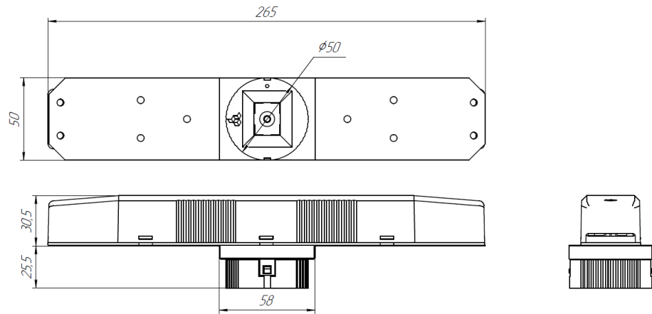
Рис. №2 Габаритный чертёж. BS-OKO-81-L1-INEXI3-AUTOTESTGR и BS-OKO-81-L2-INEXI3-AUTOTEST GR
