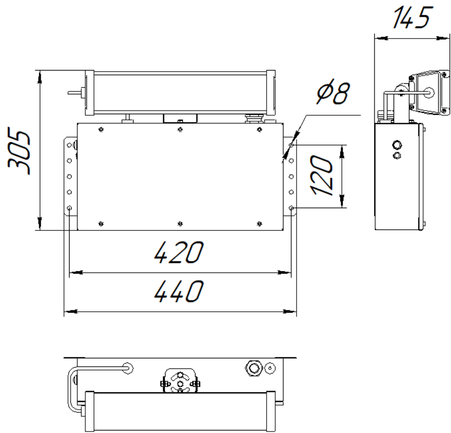
Рис. №2 Габаритный чертёж.
