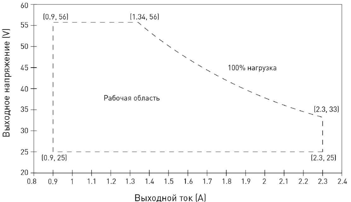
График рабочей области ограниченный максимальной мощностью (линия АБ).
