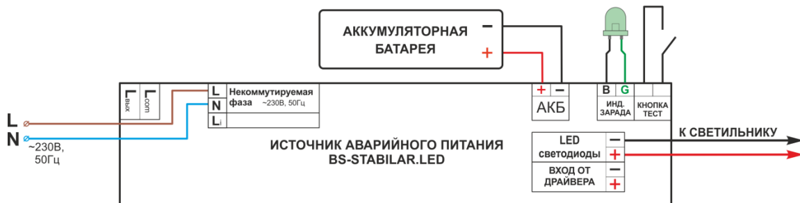
Рис. 2 Схема подключения BS-STABILAR-81-B4-LED и BS-STABILAR-83-B4-LED для аварийного светового прибора в непостоянном режиме:
