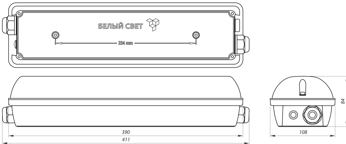
Рис.7 Габаритные и присоединительные размеры источника аварийного питания STABILAR.LED
