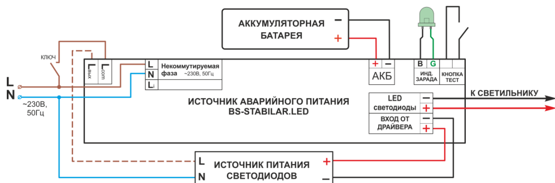
Рис. 1 Схема подключения BS-STABILAR-81-B4-LED и BS-STABILAR-83-B4-LED для аварийного светового прибора в универсальном режиме:
